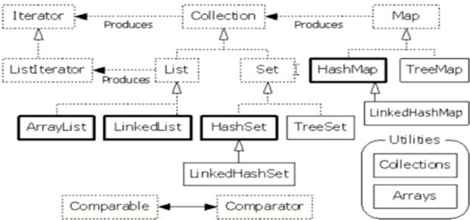
java 中集合类的关系图
